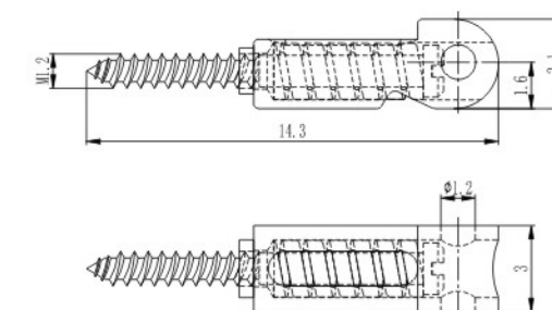
弹簧芯子 Spring core
