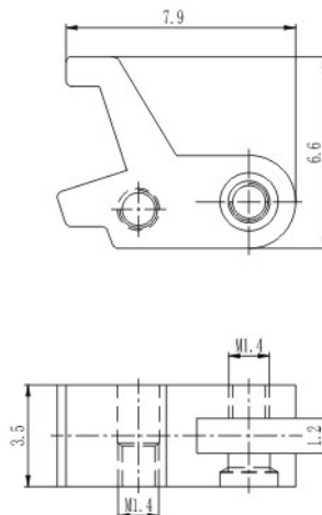
庄头 Lug XC3536-35/WG01
