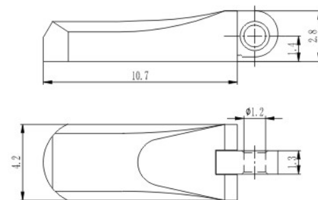
组合弹簧盒 Spring hinge
