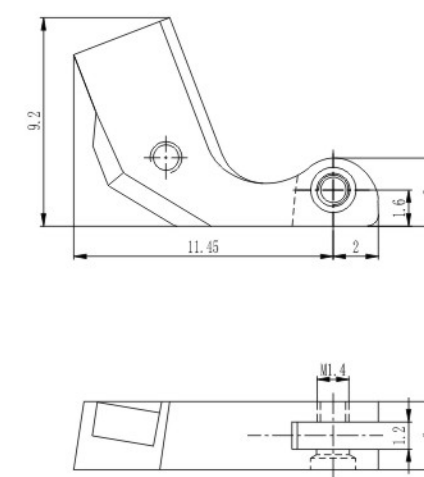
庄头 Lug XCP4034-30-Y 材料/Material: 无铅白铜/Lead free nickel silver
