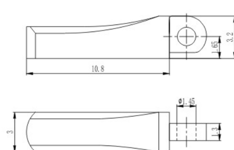
组合弹簧盒 Spring hinge
