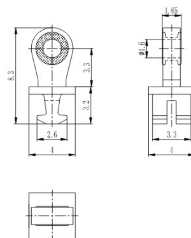
加胶铰链 Safely hinge XAD015F40-WN
