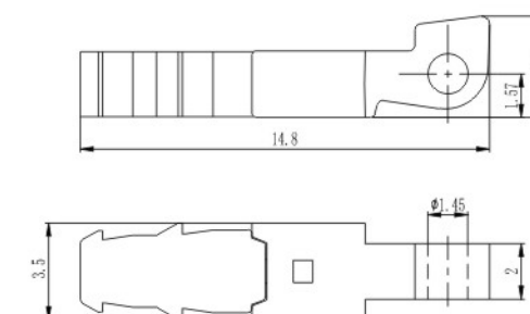
弹簧芯子 Spring core
