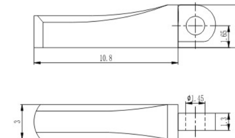
组合弹簧盒 Spring hinge
