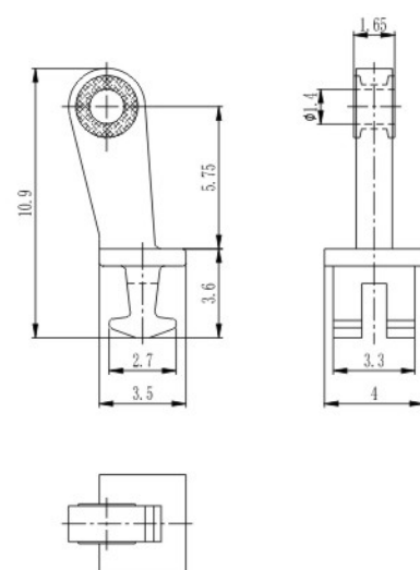
加胶铰链 Safely hinge XAD4031-40-WN
