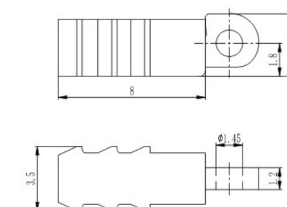
组合弹簧盒 Spring hinge
